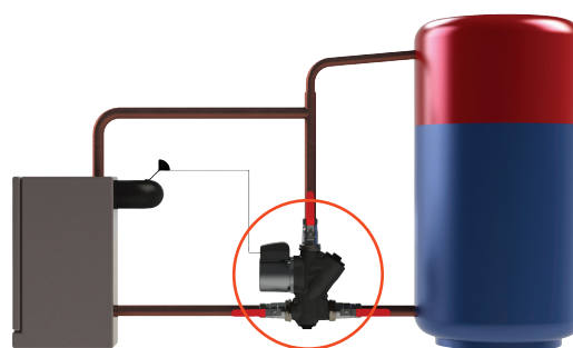
Laddomat 21 placerad mellan panna och tank.
